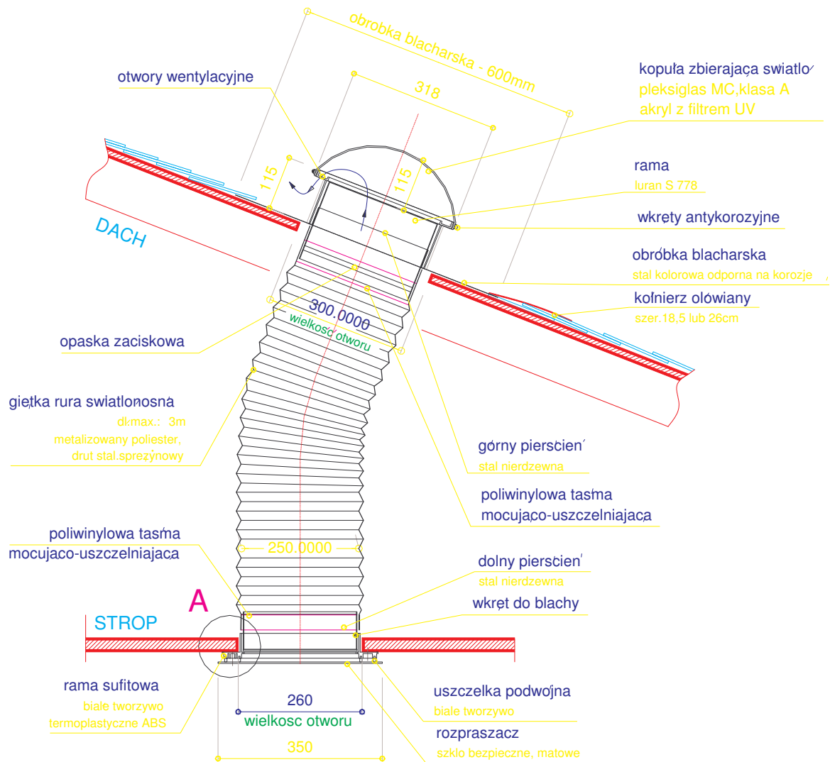
Schemat zestawieniowy elementów świetlika rurowego maxiSolar® small
